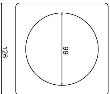
Lunetta quadrata Square bezel
