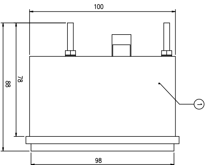
Lunetta rotonda Round bezel
